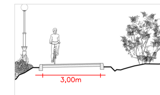
DETALHE PISTA DE CAMINHADA
